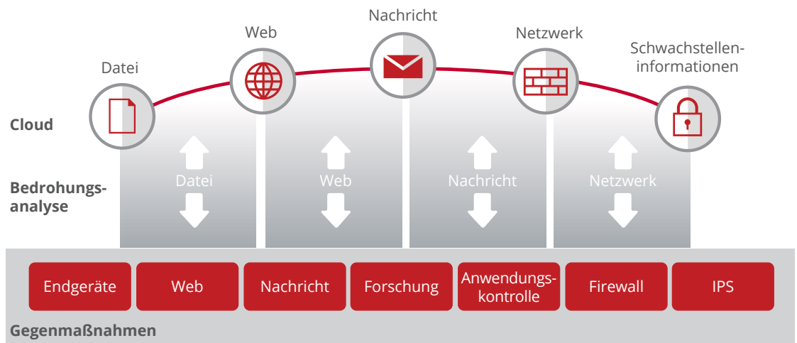
Abbildung 1. McAfee Global Threat Intelligence-Framework
