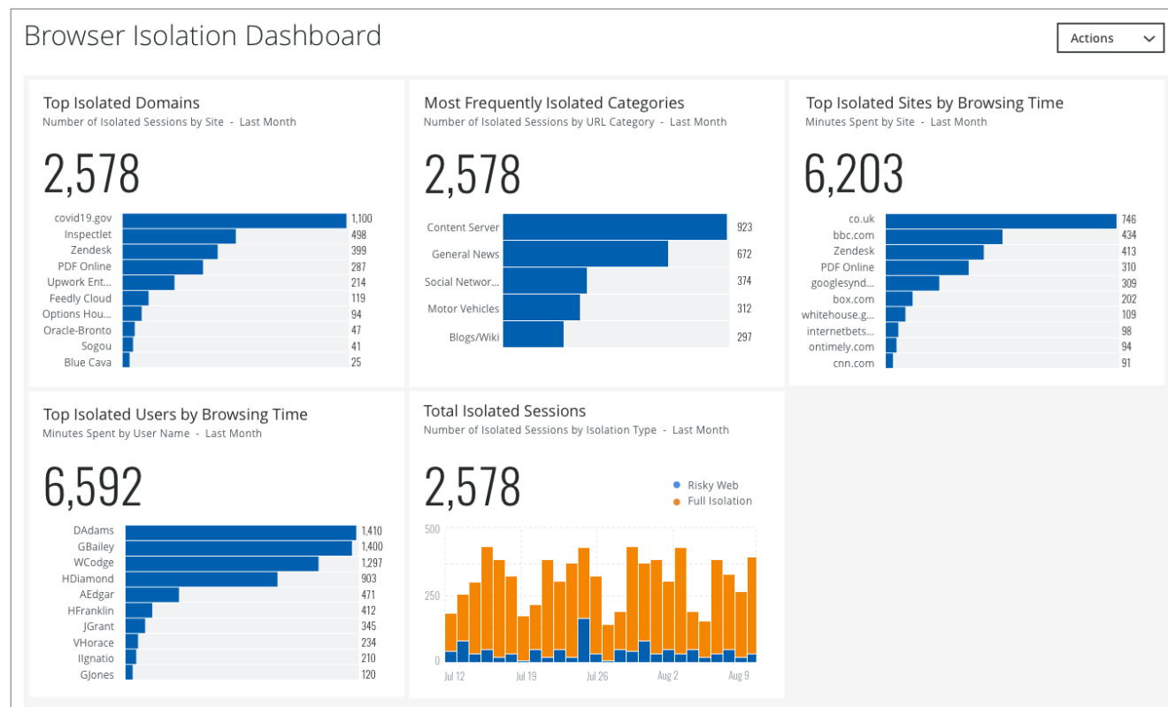
Figura 2. Interfaz de administración de McAfee Remote Browser Isolation.
