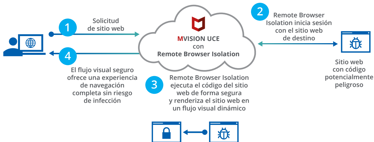
Figura 1. Funcionamiento de McAfee Remote Browser Isolation.
