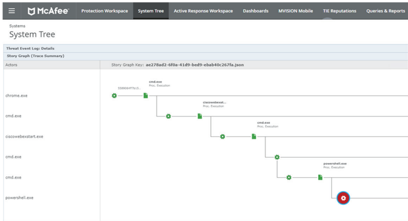
图 2. Story Graph。
