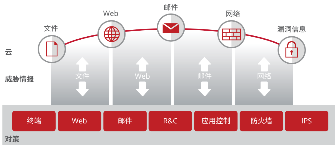
图 1. McAfee Global Threat Intelligence 框架。
