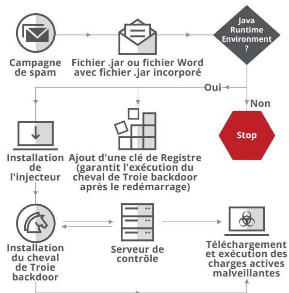
Figure 2. Chaîne d'infection d'Adwind
