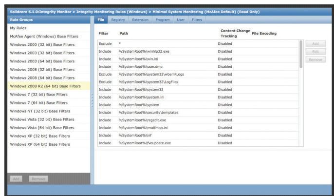
Рис. 1. McAfee Change Control содержит готовые правила мониторинга целостности файлов и продуманный набор фильтров, позволяющих следить только за теми файлами, которые вам необходимы.
