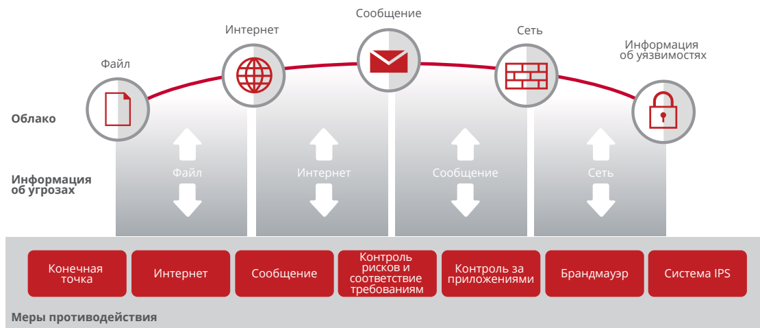
Рис. 1. Система McAfee Global Threat Intelligence
